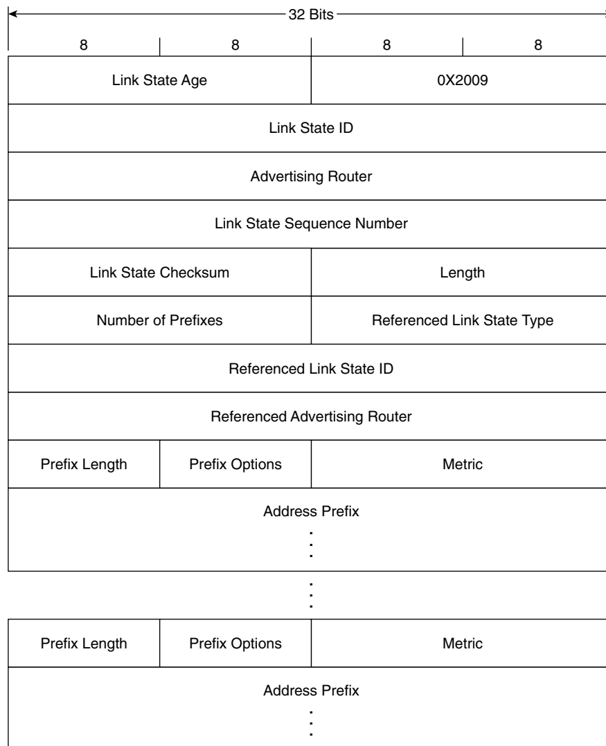
Figure 9-13 Intra-Area Prefix LSA.
