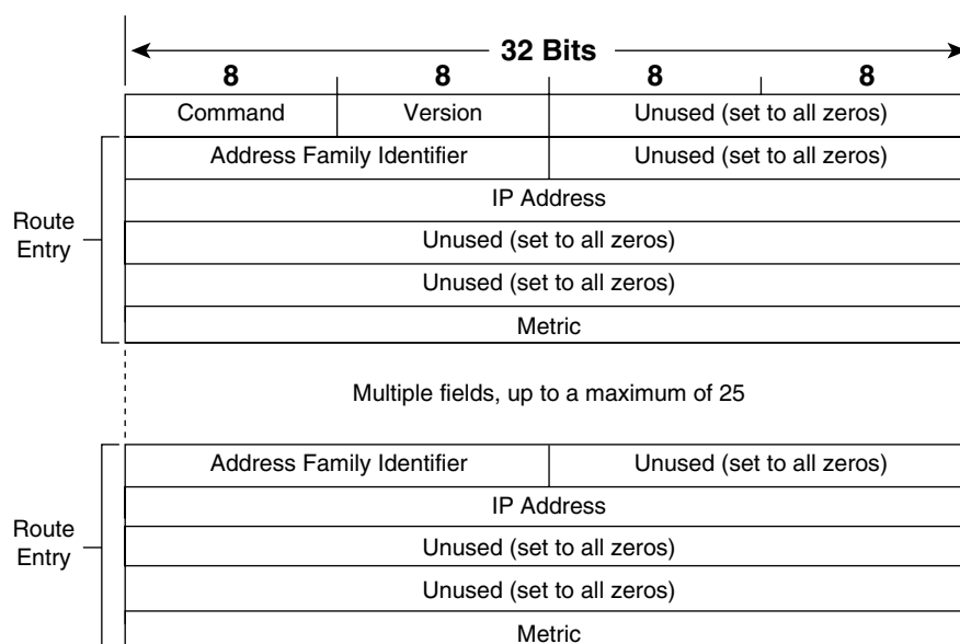
Figure 5-2 The RIP message format.
