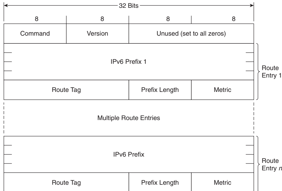
Figure 6-10 The RIPng message format.
