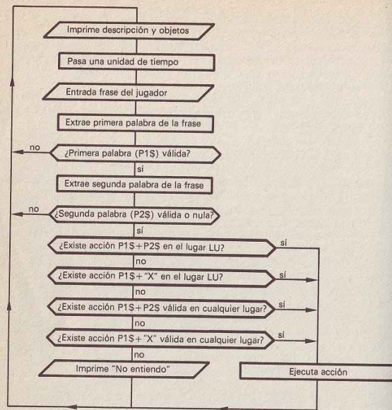
Figura 1.—Diagrama de flujo simplificado del analizador sintáctico.
