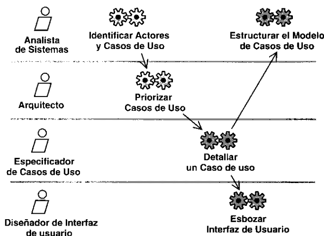
Figura 2.6. Un flujo de trabajo con trabajadores y actividades en “calles”.
