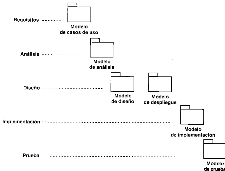
Figura 3.1. El Proceso Unificado consiste en una serie de flujos de trabajo que van desde los requisitos hasta las pruebas (de izquierda a derecha y de arriba hacia abajo). Los flujos de trabajo desarrollan modelos, desde el modelo de casos de uso hasta el modelo de prueba.
