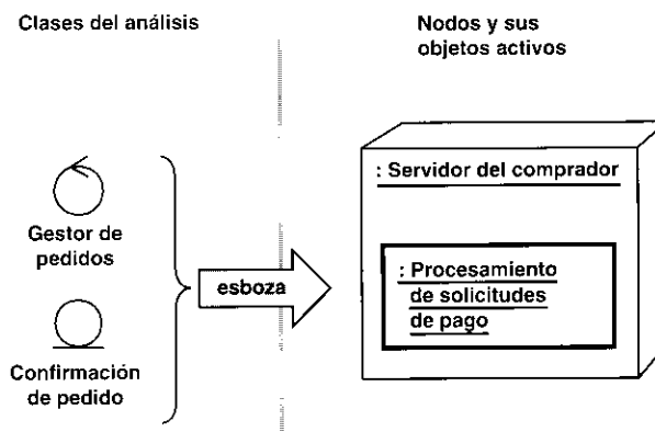
Figura 9.30. Una clase activa, procesamiento de solicitudes de pago, obtenida mediante el estudio de las clases del análisis Gestor de Pedidos y Confirmación de Pedido y del nodo Servidor del Comprador. Se decidió que las principales partes de las clases del diseño correspondientes se ubicarían en el nodo servidor del Comprador. Después se identificó la clase Procesamiento de Solicitudes de Pago para encapsular el hilo de control de esas clases del diseño dentro del nodo.
