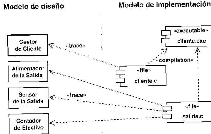
Figura 3.12. Componentes que implementan clases de diseño.
