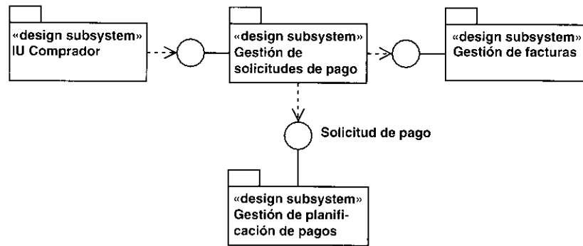
Figura 9.38. Diagrama de clases con subsistemas, interfaces, y sus dependencias.
