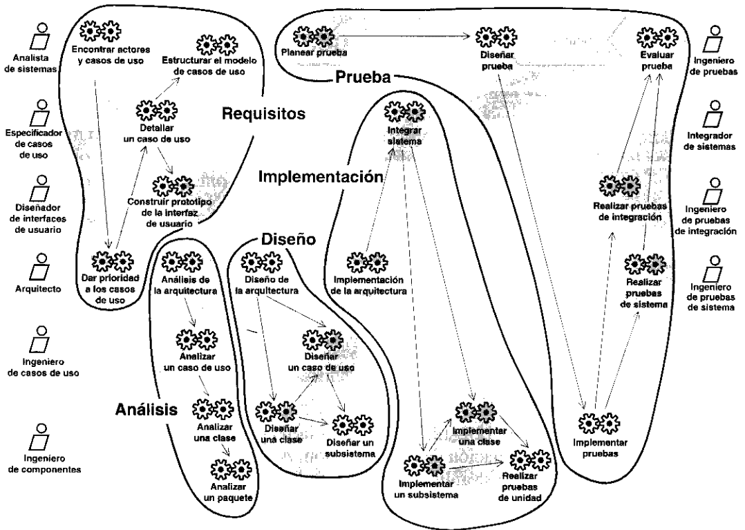
Figura 12.3. Los nombres de los trabajadores están colocados en los márgenes izquierdo y derecho, identificando las “calles”. El tiempo avanza de izquierda a derecha. Los flujos de trabajo, incluyendo los trabajadores y las actividades que realizan, están representados por los “círculos” de trazo libre. El ingeniero de componentes, por ejemplo, diseña una clase y un subsistema en el flujo de diseño, implementa una clase y un subsistema y realiza una prueba de unidad en el flujo de implementación.
