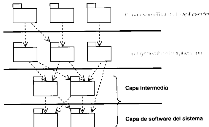
Figura 9.24. Los subsistemas de las capas intermedia y de software del sistema encapsulan productos software comprados.
