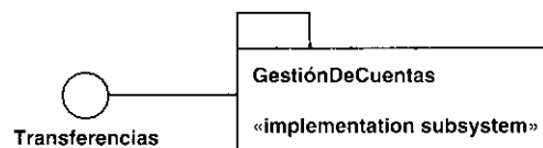
Figura 10.10. El subsistema GestiónDeCuentas proporciona la interfaz Transferencias.
