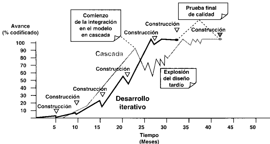
Figura 5.2. En el método en cascada (la línea fina), los desarrolladores no comienzan la implementación hasta haber terminado los requisitos, y el diseño. Informan de un buen progreso en la implementación porque no tienen construcciones intermedias que les indiquen otra cosa. Los problemas están aún ocultos bajo tierra hasta que la integración y las pruebas los descubran todos a la vez (Explosión del Diseño Tardío). En el desarrollo iterativo, la implementación comienza más al principio y las construcciones frecuentes no sólo descubren pronto los problemas, sino que también los solucionan en pequeños lotes más fáciles de manejar.
