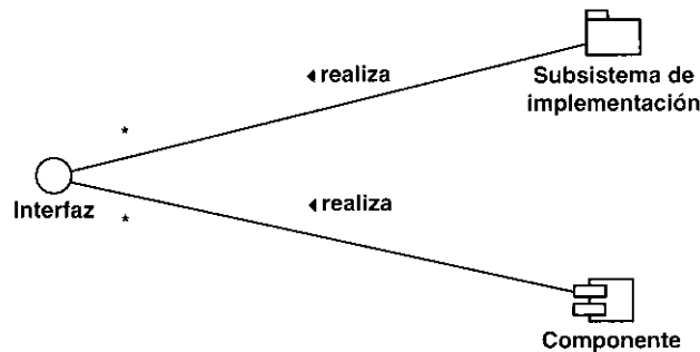
Figura 10.9. Las asociaciones fundamentales de una interfaz.
