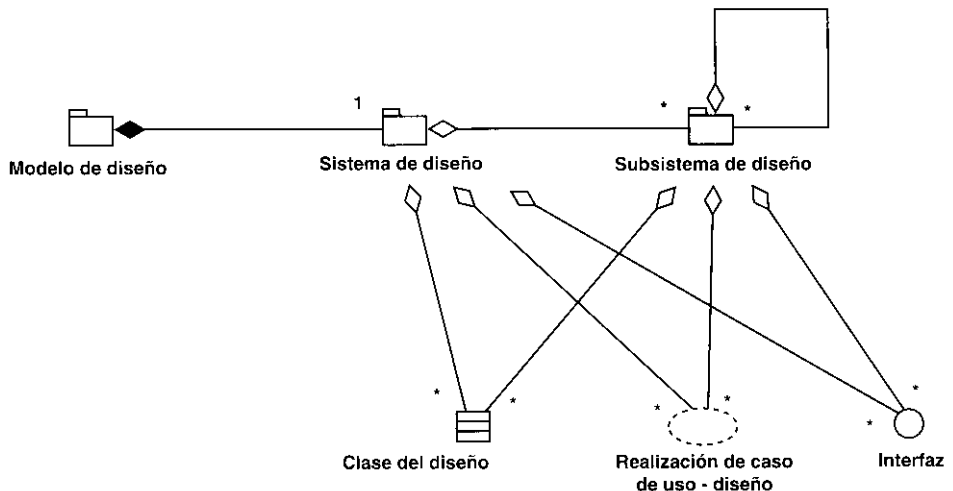
Figura 9.3. El modelo de diseño es un jerarquía de subsistemas de diseño que contienen clases del diseño, realizaciones de caso de uso-diseño e interfaces.
