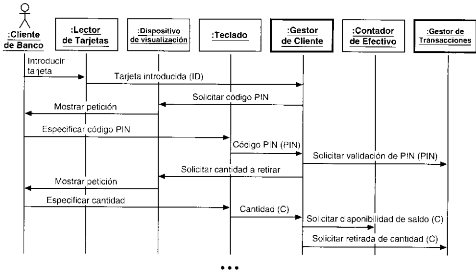
Figura 3.10. Un diagrama de secuencia que es parte de la realización del caso de uso Sacar Dinero en el modelo de diseño.
