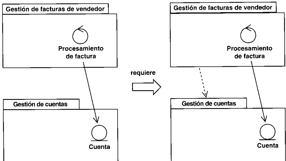
Figura 8.30. Dependencias necesarias entre paquetes.
