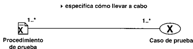
Figura 11.5. Hay asociaciones muchos-a-muchos entre los procedimientos de prueba y los casos de prueba.
