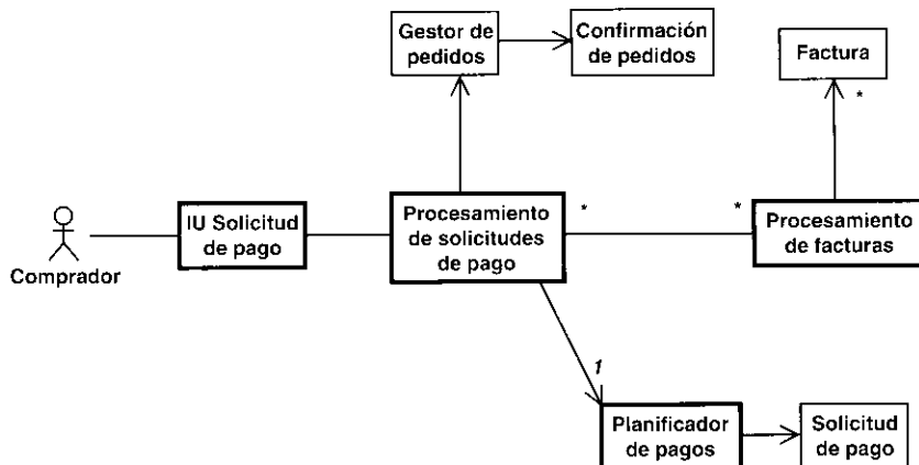
Figura 9.35. Las clases que participan en la realización del caso de uso Pagar Factura y sus asociaciones. En el diagrama, mostramos las clases activas con bordes más gruesos.
