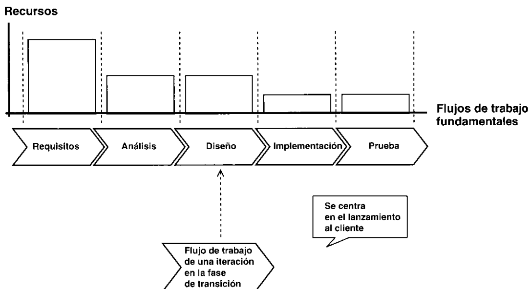
Figura 16.1. El trabajo de una iteración durante la fase de transición discurre a lo largo de los mismos cinco flujos de trabajo que las fases anteriores. (El tamaño de las barras tiene un carácter meramente ilustrativo, y será distinto en diferentes proyectos.) Los flujos de trabajo de implementación y pruebas son los que reciben mayor atención en esta fase. Es aquí donde los defectos encontrados durante las pruebas beta o las de aceptación se identifican, corrigen y prueban de nuevo. En unos pocos casos será necesario rediseñar, para corregir los defectos, lo que llevaría a un pequeño aumento en el flujo de trabajo de diseño. Los requisitos no se ven muy afectados.
