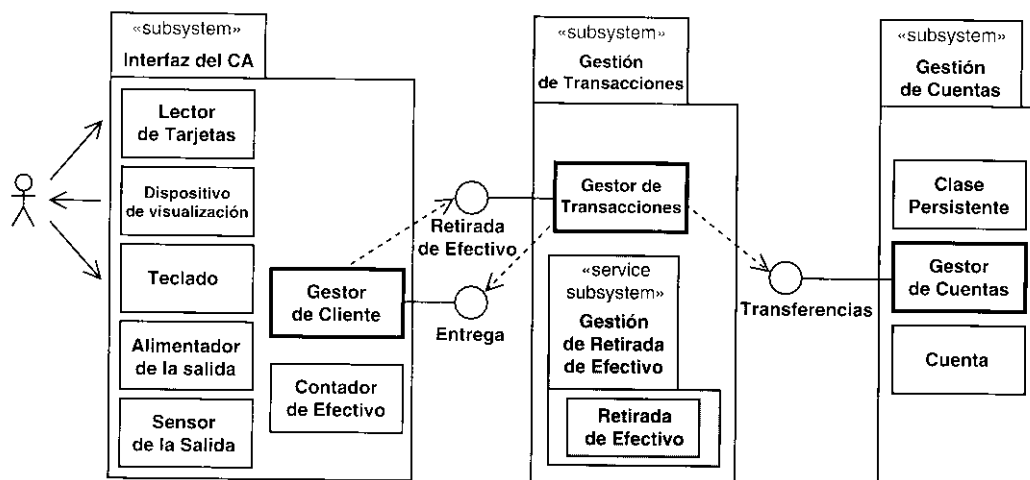
Figura 3.11. Tres subsistemas y un subsistema de servicio (en gris dentro del subsistema de Gestión de Transacciones) para nuestro ejemplo sencillo del CA.
