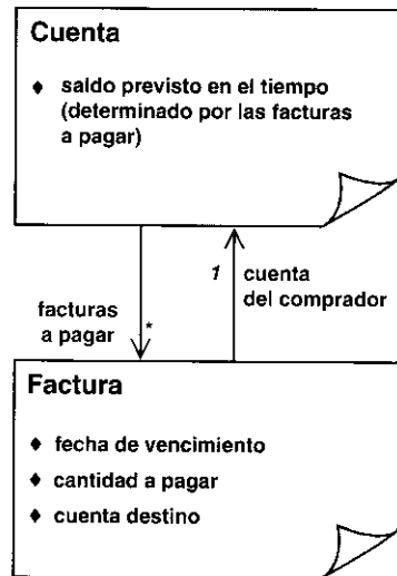
Figura 7.18. Elementos de la interfaz de usuario para Cuenta y Factura, con algunos de sus atributos indicados.
