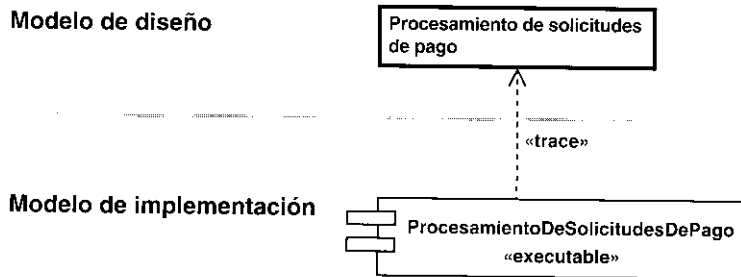
Figura 10.18. Las clases activas se usan para identificar componentes ejecutables.
