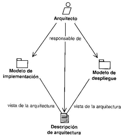
Figura 10.13. Las responsabilidades del arquitecto en la implementación.
