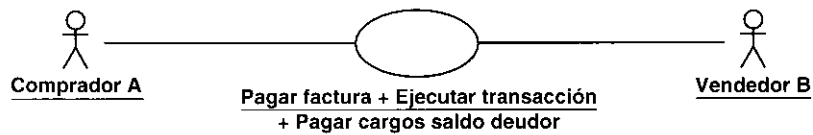
Figura 7.24. La instancia del caso de uso real formado por los casos de uso Pagar Factura y Ejecutar Transacción extendidos mediante el caso de uso Pagar Cargos Saldo Deudor, tal y como lo perciben las instancias de los actores Comprador A y Vendedor B.
