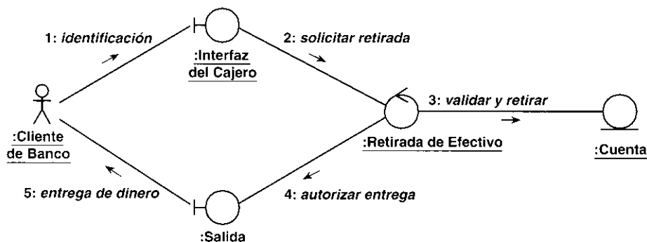
Figura 3.6. Un diagrama de colaboración para la realización del caso de uso Sacar Dinero en el modelo de análisis.
