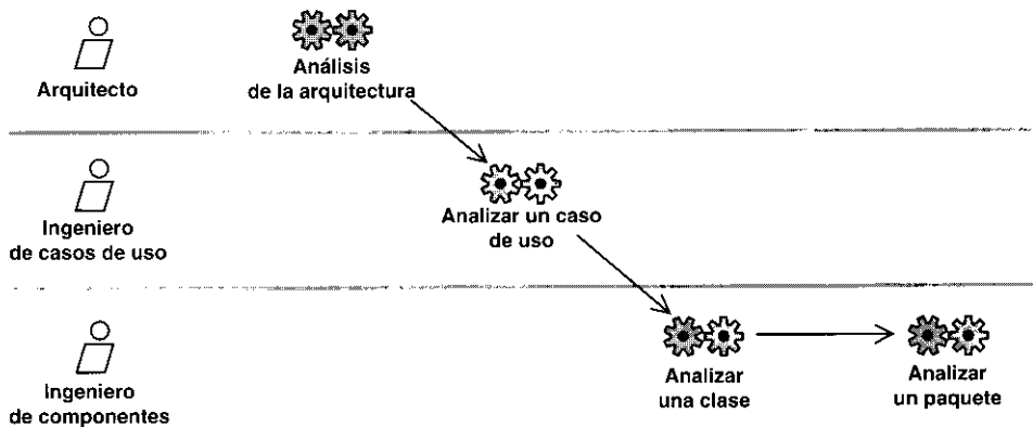
Figura 8.18. El flujo de trabajo en el análisis, incluyendo a los trabajadores participantes y sus actividades.
