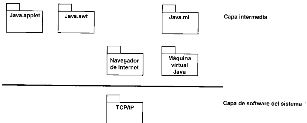
Figura 9.25. La capa intermedia de Java proporciona interfaces gráficos de usuario independientes de la plataforma ( java.awt ) y distribución de objetos ( java.rmi ). Esta figura no muestra ninguna dependencia entre subsistemas (las presentaremos en la Figura 9.26).
