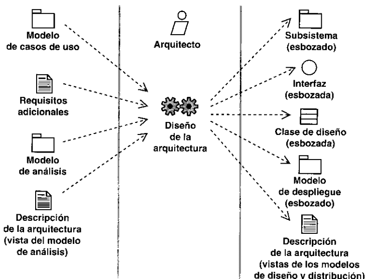
Figura 9.17. Las entradas y los resultados del diseño de la arquitectura.
