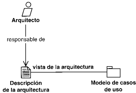
Figura 7.9. Las responsabilidades de un arquitecto durante la captura de requisitos en forma de casos de uso.
