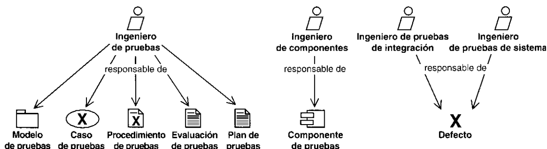
Figura 11.1. Los trabajadores y artefactos involucrados en las pruebas.
