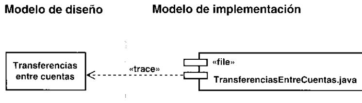
Figura 10.4. Dependencias de traza entre componentes y clases de diseño.
