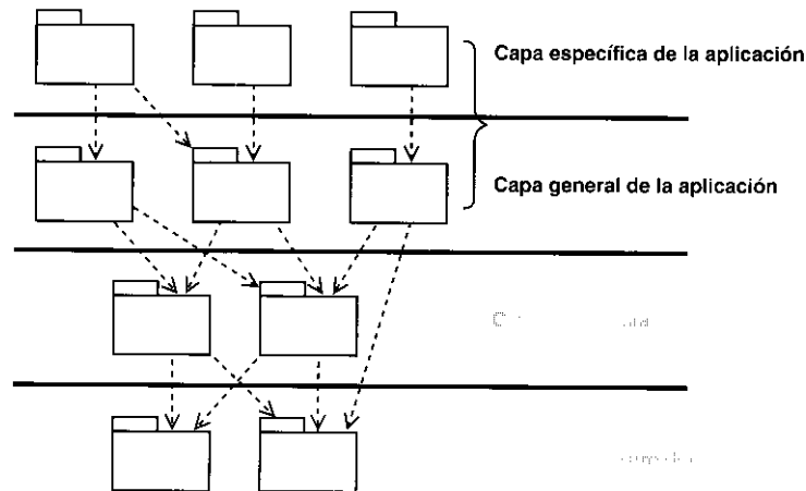
Figura 9.19. Subsistemas en las capas específica de la aplicación y general de la aplicación.
