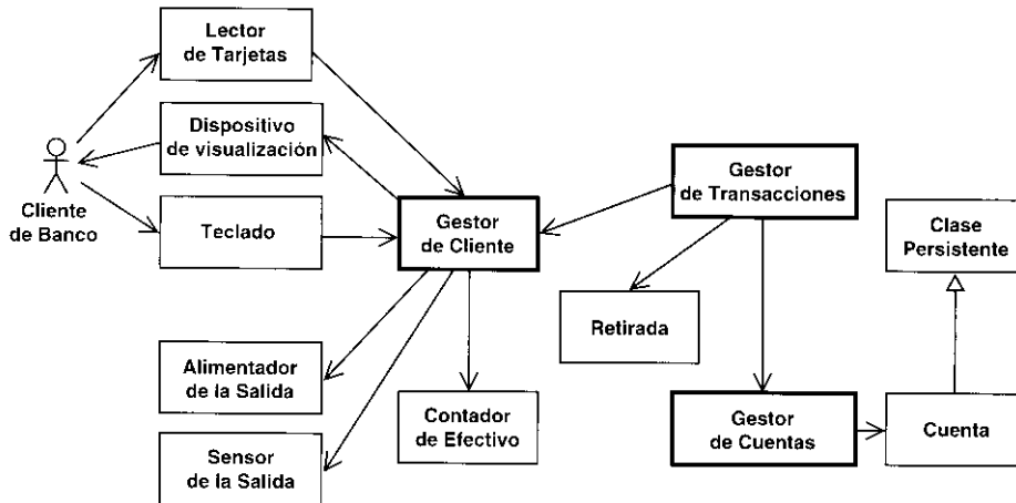
Figura 3.9. Un diagrama de clases que es parte de la realización del caso de uso Sacar Dinero en el modelo de diseño. Cada clase de diseño participa y asume roles en la realización del caso de uso.
