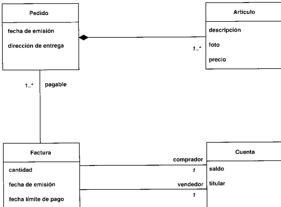
Figura 6.3. Un diagrama de clases en un modelo del dominio, que captura los conceptos más importantes del contexto del sistema.
