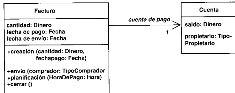
Figura 9.5. La clase de diseño Factura con sus atributos, operaciones y una asociación que asocia los objetos Factura con los objetos Cuenta.
