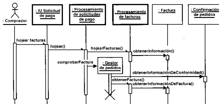
Figura 11.11. Primera parte de un diagrama de secuencia para la realización de caso de uso-diseño del caso de uso Pagar Factura.
