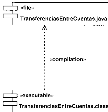
Figura 10.6. Dependencias de compilación entre dos componentes.
