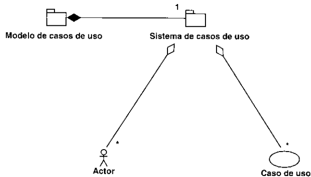
Figura 7.2. El modelo de casos de uso y sus contenidos. El sistema de casos de uso representa el paquete de más alto nivel del modelo.
