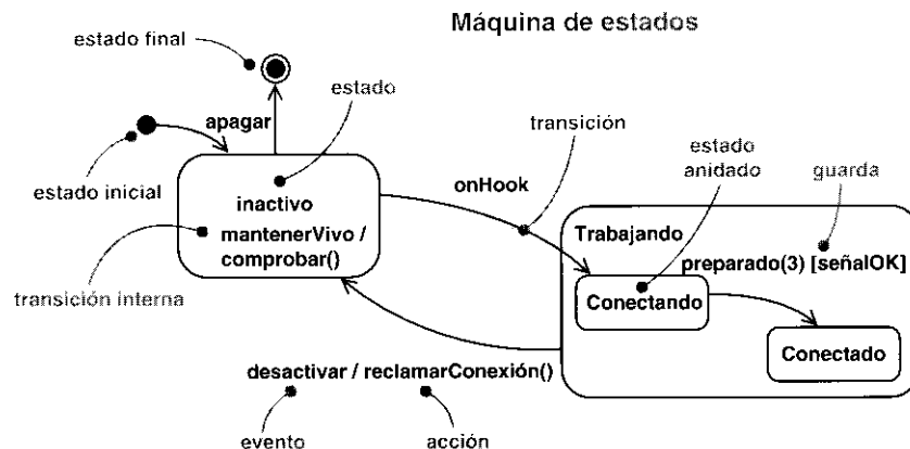
Figura A.6. Máquinas de estados.
