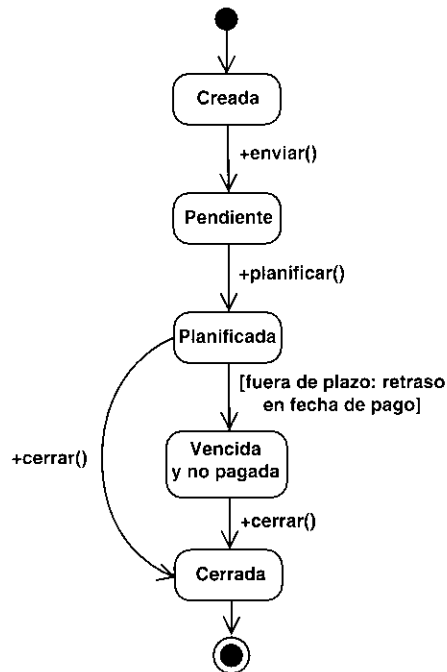
Figura 9.42. Un diagrama de estados para la clase Factura.
