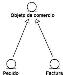
Figura 8.28. Objeto de comercio generaliza factura y pedido.
