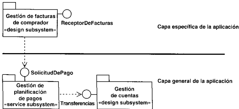
Figura 9.28. Las interfaces en las dos capas superiores del modelo de diseño.
