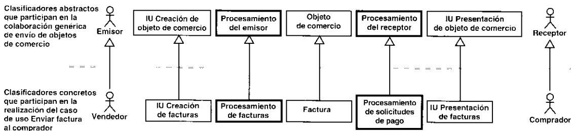
Figura 9.33. Clasificadores concretos participantes en una determinada realización de caso de uso que son subtipos de los clasificadores abstractos que participan en una colaboración genérica.
