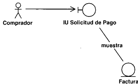
Figura 8.7. La clase de entidad Factura y su relación con la clase de interfaz IU Solicitud de Pago.
