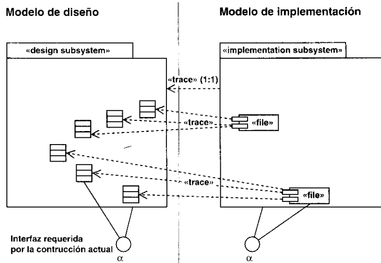
Figura 10.23. Una interfaz requerida en una construcción ( \alpha ) debería ser proporcionada también por un subsistema de implementación.
