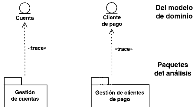
Figura 8.21. Identificación de paquetes del análisis generales a partir de clases del dominio.
