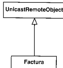
Figura 9.43. Los objetos de la clase Factura deben estar distribuidos. Esto se realiza convirtiéndolos en subtipos de UnicastRemoteObjects .
