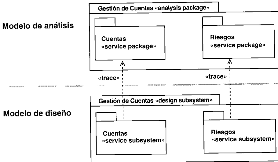
Figura 9.21. Identificación de subsistemas de servicio a partir de paquetes de servicio existentes.
