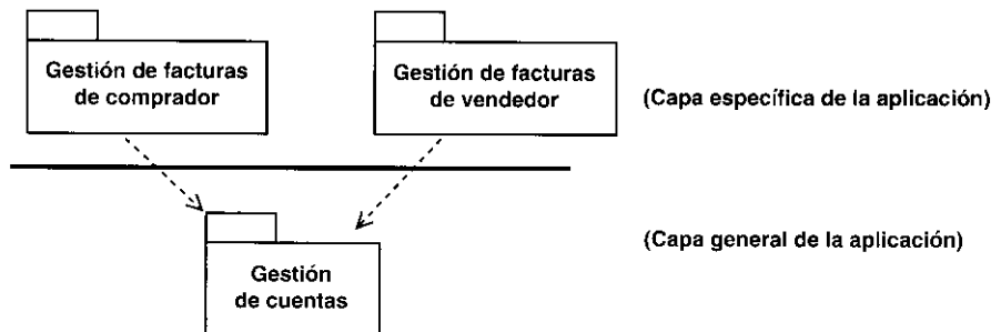
Figura 8.24. Dependencias y capas de paquetes del análisis.
