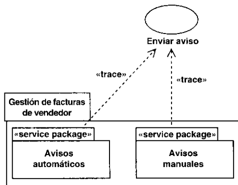
Figura 8.22. Los paquetes de servicio, Avisos automáticos y Avisos manuales, ubicados dentro del paquete Gestión de Facturas de Vendedor.
