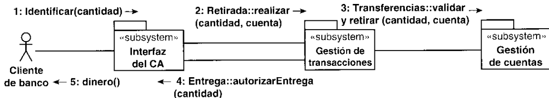
Figura 4.9. Los subsistemas que colaboran en la ejecución del caso de uso Sacar Dinero.
