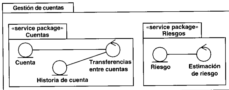
Figura 8.23. Los paquetes de servicio Cuentas y Riesgos, cada uno de ellos encapsulando clases relacionadas funcionalmente.
