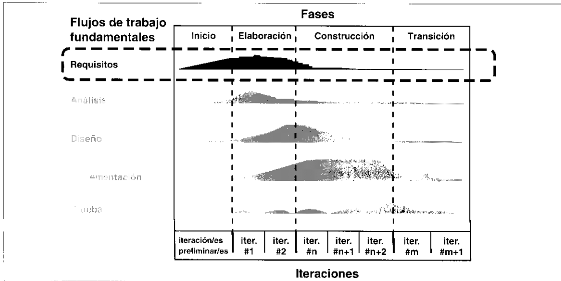
Figura 6.2. El trabajo de los requisitos se hace fundamentalmente durante el inicio y la elaboración.
