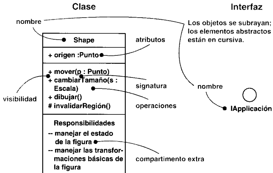
Figura A.2. Clases e interfaces.
