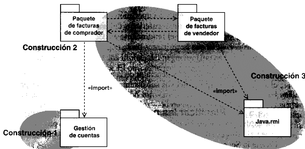
Figura 14.3. La primera iteración se compone de tres construcciones. Obsérvese que la Construcción 2 incluye también los resultados de la Construcción 1.
