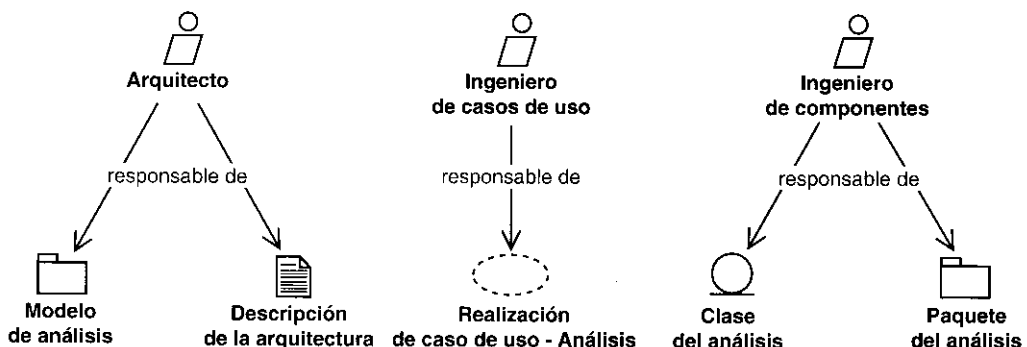
Figura 8.1. Los trabajadores y artefactos implicados en el análisis.
