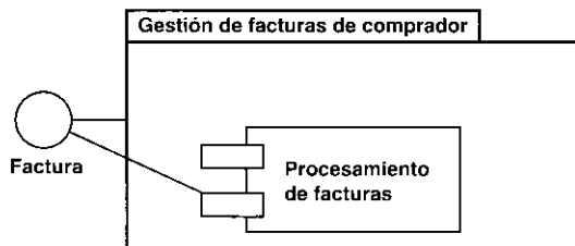
Figura 10.24. El componente Procesamiento de Facturas proporciona la interfaz Facturas.
