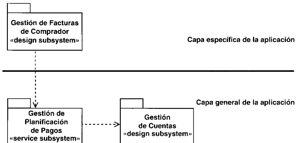
Figura 9.22. Durante el diseño, se identificó el subsistema de servicio Gestión de Planificación de Pagos para proporcionar un servicio general que puedan utilizar diferentes realizaciones de casos de uso.
