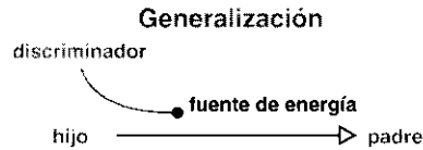
Figura A.11. Relaciones de generalización.
