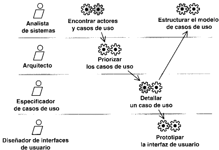
Figura 7.10. El flujo de trabajo para la captura de requisitos en forma de casos de uso, incluyendo trabajadores participantes y sus actividades.
