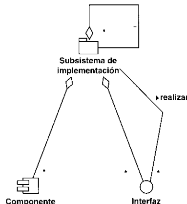
Figura 10.7. Contenido y asociaciones clave de un subsistema.
