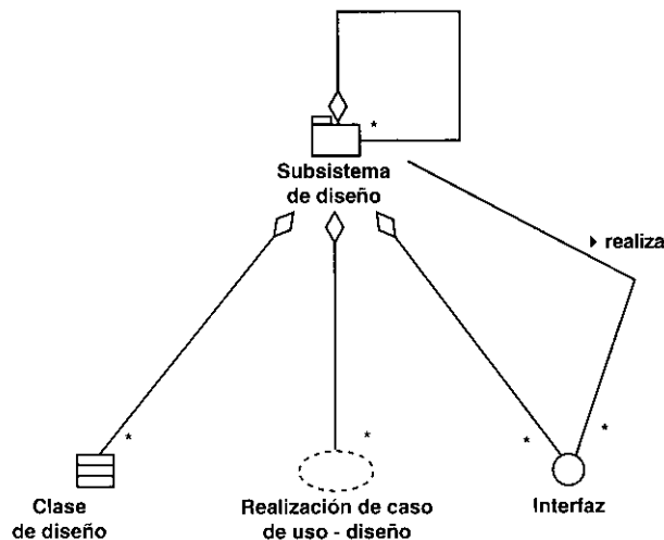
Figura 9.8. Los contenidos de un subsistema y sus asociaciones fundamentales.
