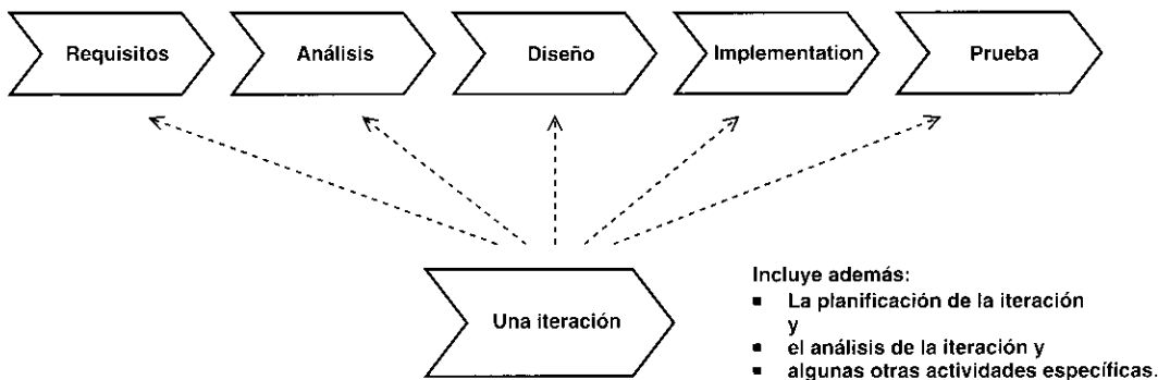
Figura 5.3. Cada iteración constituye una pasada a través de los cinco flujos de trabajo fundamentales. Se inicia con una actividad de planificación y se concluye con un análisis.
