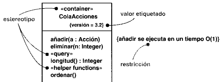
Figura A.12. Mecanismos de extensibilidad.
