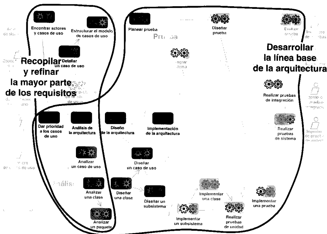
Figura 14.2. En esta figura se resaltan las actividades principales de la fase de elaboración.
