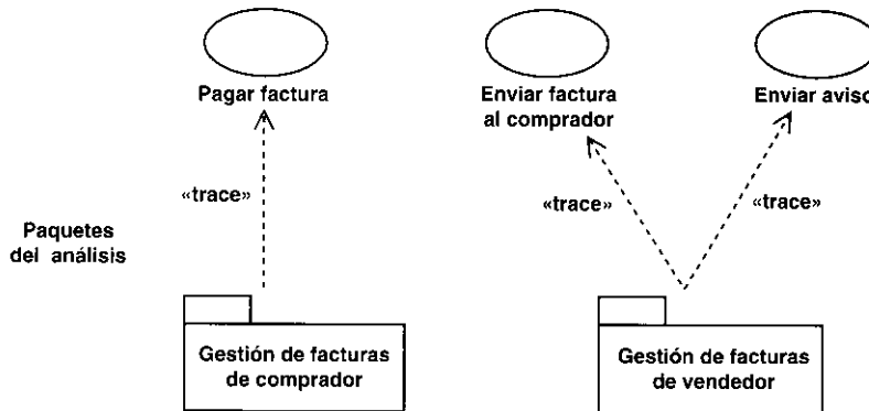
Figura 8.20. Identificación de paquetes del análisis a partir de los casos de uso.
