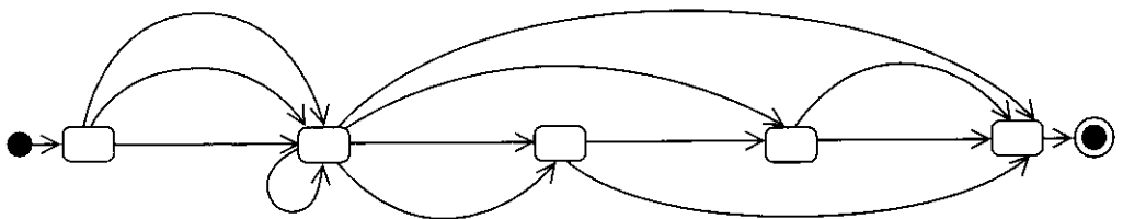
Figura 7.15. Un caso de uso puede imaginarse como si tuviera un estado de comienzo (el rectángulo redondeado de más a la izquierda), estados intermedios (los subsiguientes rectángulos redondeados), estados finales (el rectángulo redondeado de más a la derecha) y transiciones de un estado a otro. (Véase el Apéndice A para la notación de diagramas de estados.) Las flechas rectas ilustran el camino básico, y las curvas, otros caminos.
