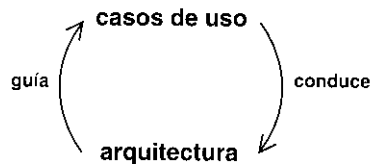
Figura 4.3. Los casos de uso conducen el desarrollo de la arquitectura, y la arquitectura indica qué casos de uso pueden realizarse.
