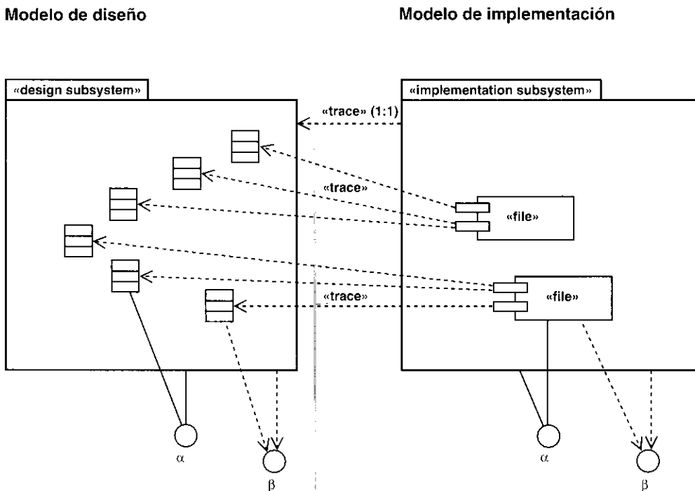
Figura 10.8. Un subsistema de implementación en el modelo de implementación que sigue la traza uno a uno a un subsistema de diseño en el modelo de diseño. Los subsistemas en los diferentes modelos proporcionan la misma interfaz ( \alpha ) y dependen de la misma interfaz ( \beta ). Los componentes en el sistema de implementación implementan clases en el subsistema de diseño.
