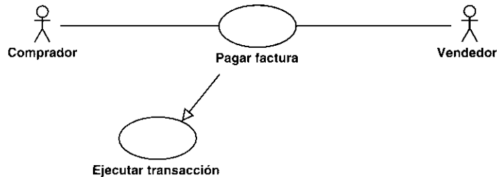
Figura 7.21. La relación de generalización entre los casos de uso Pagar Factura y Ejecutar Transacción.
