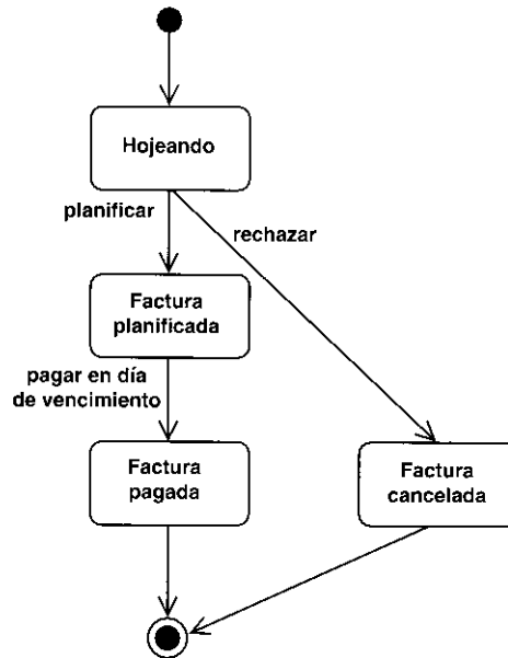
Figura 7.16. El diagrama de estados para el caso de uso Pagar Factura muestra cómo una instancia del caso de uso Pagar Factura transita por diferentes estados (rectángulos redondeados) en una secuencia de transiciones de estado (flechas).
