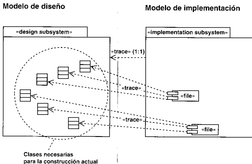
Figura 10.22. Las clases de diseño necesarias en una construcción se implementan con componentes.
