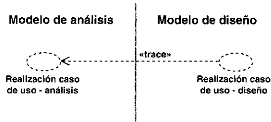
Figura 9.6. Trazas existentes entre realizaciones de caso de uso en diferentes modelos.
