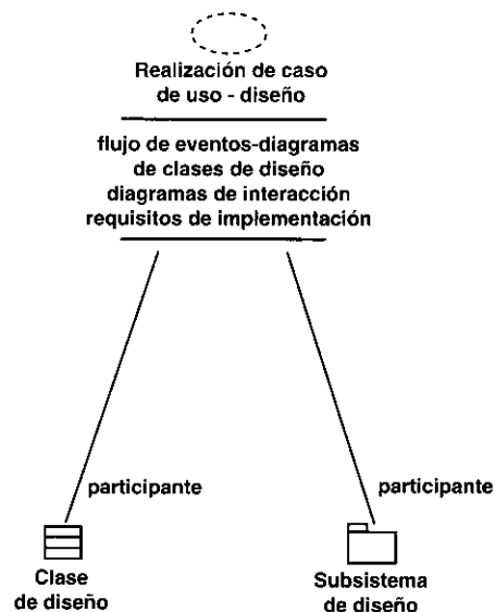
Figura 9.7. Los atributos clave y asociaciones de una realización de caso de uso-diseño.
