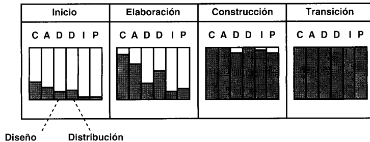
Figura 5.7. El trabajo en todos los modelos continúa en todas las fases, como se indica con el relleno creciente de los modelos. La fase de construcción finaliza con un conjunto de modelos (casi) completo. Sin embargo, estos modelos necesitan ajustes durante la transición a medida que se distribuyen en la comunidad de usuarios.
