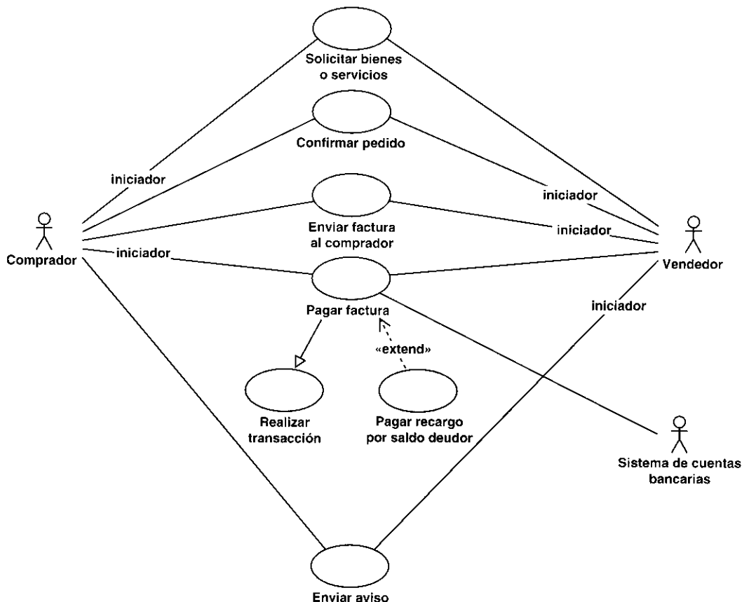
Figura 7.12. Casos de uso en el Sistema de Pagos y Facturación que soporta el caso de uso del negocio Ventas: del pedido a la entrega. El papel iniciador , conectado a las asociaciones, indica qué actor comienza el caso de uso.
