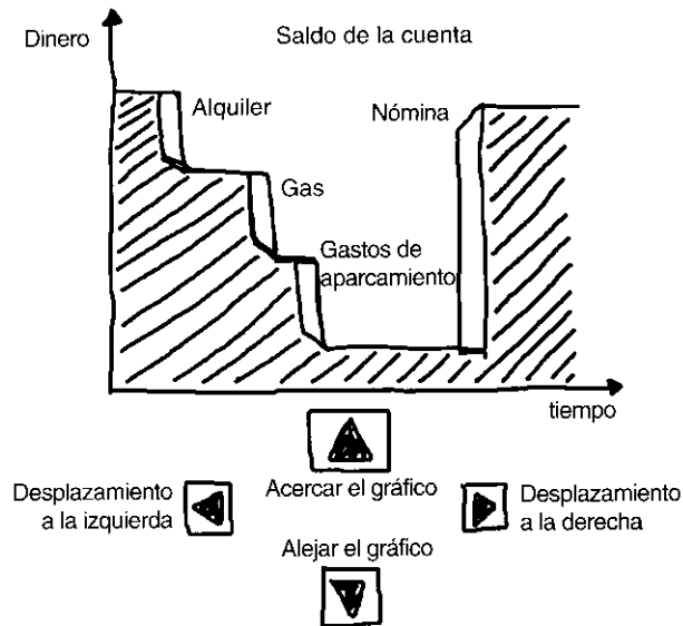
Figura 7.19. Una interfaz de usuario propuesta para los elementos de interfaz relacionados Cuenta y Factura. La interfaz muestra cómo incrementan o reducen la cuenta los pagos de facturas e ingresos de depósitos. Los botones de desplazamiento izquierdo y derecho mueven la ventana de tiempo en la que el actor puede estudiar el saldo de la cuenta. Los botones de alejar y acercar cambian la escala del diagrama.
