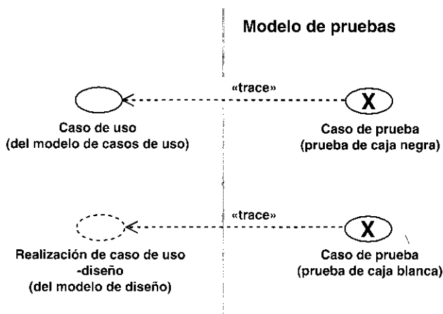
Figura 11.4. Un caso de prueba puede derivarse de, y por tanto puede seguir la traza de, un caso de uso en el modelo de casos de uso o de una realización de caso de uso en el modelo de diseño.
