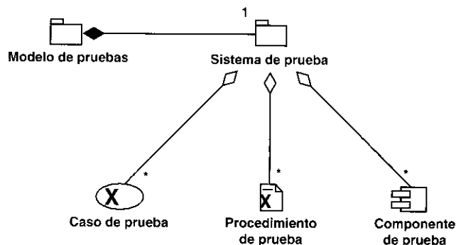
Figura 11.3. El modelo de pruebas.
