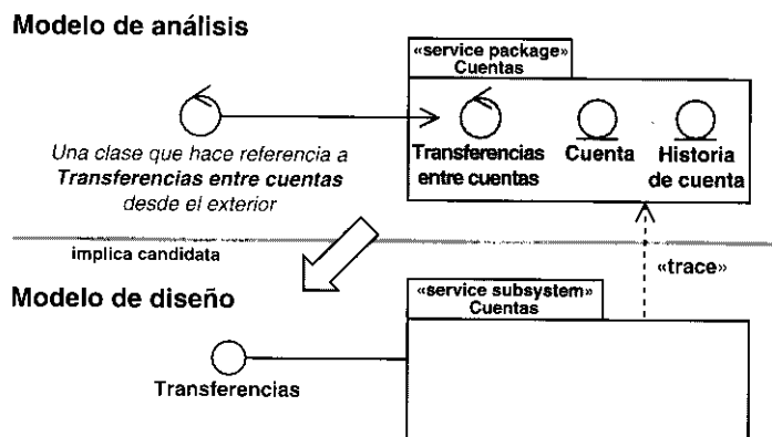
Figura 9.27. Una interfaz identificada inicialmente a partir del modelo de análisis.
