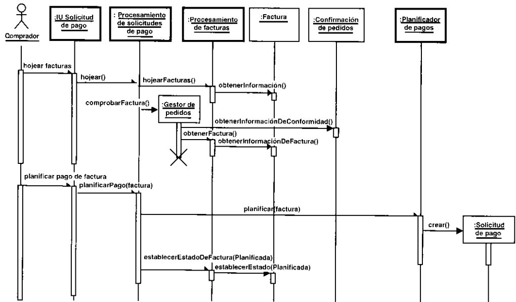
Figura 9.36. Diagrama de secuencia con los objetos de diseño que llevan a cabo parte de la realización del caso de uso Pagar Factura.
