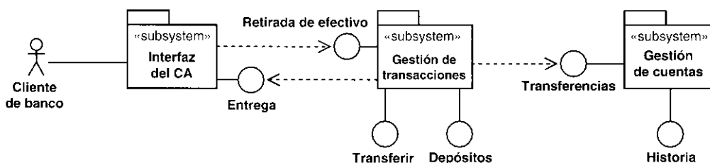
Figura 4.8. La estructura estática de la vista de la arquitectura del modelo de diseño para el sistema de CA. Este diagrama de clases muestra los subsistemas y las interfaces entre ellos.
