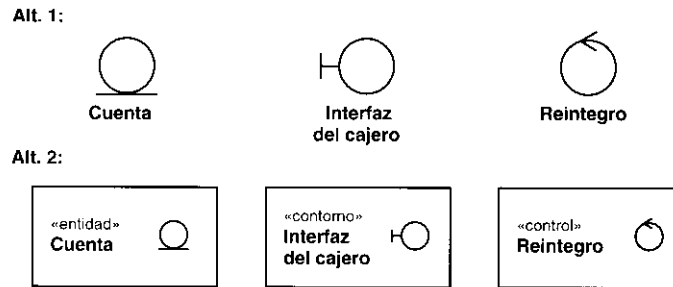
Figura B.1. Los tres estereotipos de clase estándar usados en el análisis.
