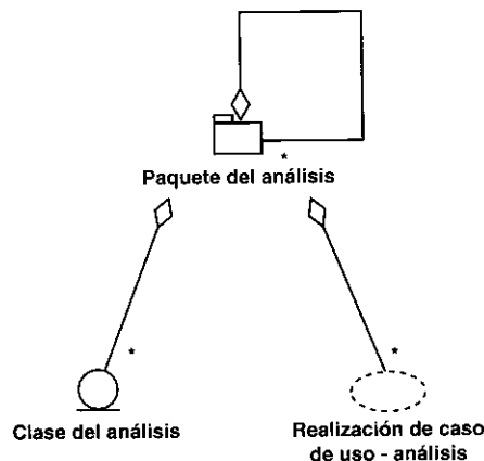
Figura 8.13. Contenidos de un paquete del análisis.
