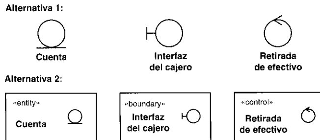
Figura 8.5. UML proporciona tres estereotipos de clases estándar que podemos utilizar en el análisis.
