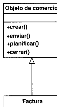
Figura 9.40. La clase Factura, su supertipo Objeto de Comercio, y las operaciones que soporta.
