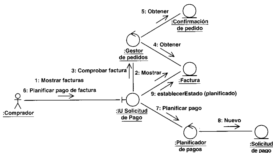
Figura 8.12. Un diagrama de colaboración de una realización del caso de uso Pagar Factura.
