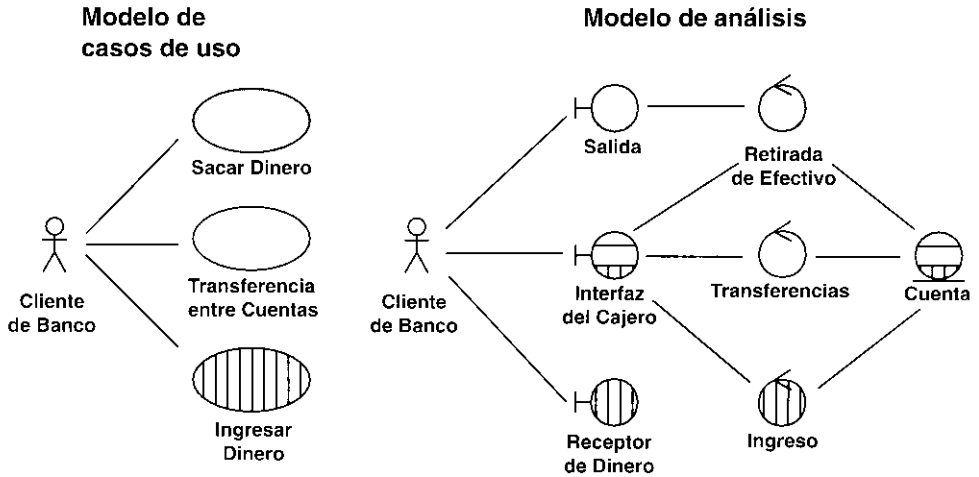
Figura 3.5. El diagrama muestra cómo cada caso de uso (izquierda) se realiza como una estructura de clases del análisis (derecha). Por ejemplo, las clases Interfaz del Cajero, Retirada de Efectivo, Cuenta y Salida participan en la realización del caso de uso Sacar Dinero. Las clases Interfaz del Cajero y Cuenta participan y desempeñan roles en las tres realizaciones de caso de uso. Las otras clases participan en una sola realización de caso de uso, es decir, desempeñan un solo rol.
