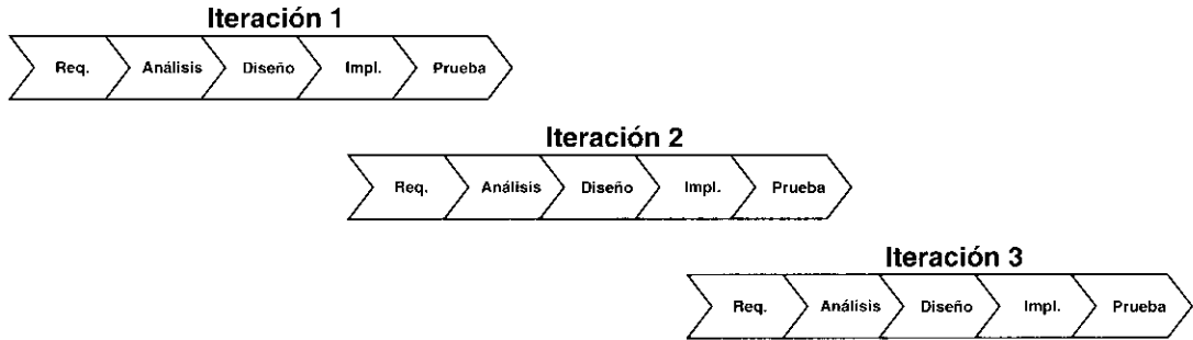
Figura 5.4. Las iteraciones discurren a lo largo de los flujos de trabajo desde la captura de requisitos hasta la prueba.
