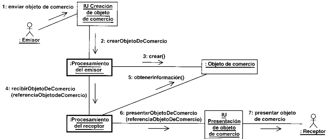
Figura 9.32. Diagrama de colaboración que ejemplifica una colaboración genérica para crear, enviar, recibir y presentar objetos de comercio.
