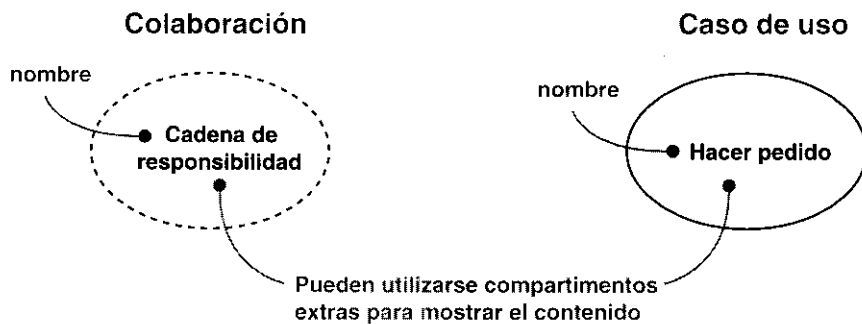
Figura A.3. Casos de uso y colaboraciones. (Obsérvese que los nombres de, por ejemplo, los casos de uso pueden ponerse fuera del símbolo si es conveniente.)
