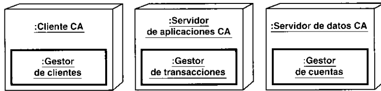
Figura 4.11. La vista arquitectónica del modelo de despliegue. Las clases activas del sistema de CA se distribuyen sobre los nodos. Los objetos activos se muestran mediante rectángulos con bordes gruesos.
