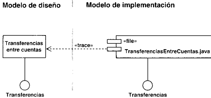
Figura 10.5. Los componentes proporcionan las mismas interfaces que las clases que implementan.
