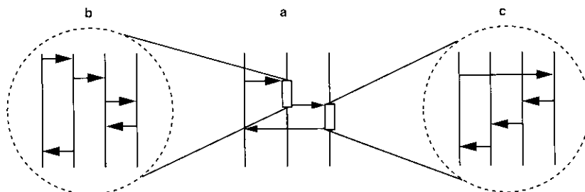
Figura 9.37. Las líneas de vida en el centro del diagrama (a) representan subsistemas, y muestran los mensajes que se envían y reciben entre subsistemas. Los otros diagramas (b, c) representan el diseño interno de los subsistemas, y muestran cómo esos mensajes (los que se muestran en a) los reciben y envían los elementos internos de los subsistemas. El diagrama (a) puede ser diseñado antes que los diagramas (b y c).
