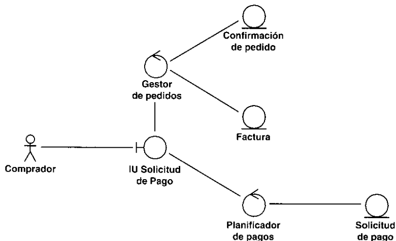
Figura 8.11. Un diagrama de clases de una realización del caso de uso Pagar Factura.
