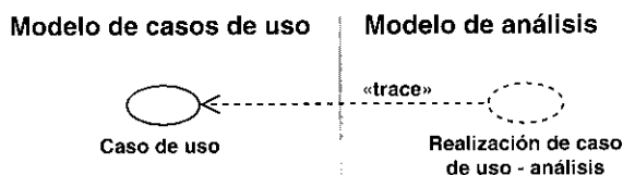
Figura 8.9. Existe una traza entre una realización de caso de uso-análisis en el modelo de análisis y un caso de uso en el modelo de casos de uso.
