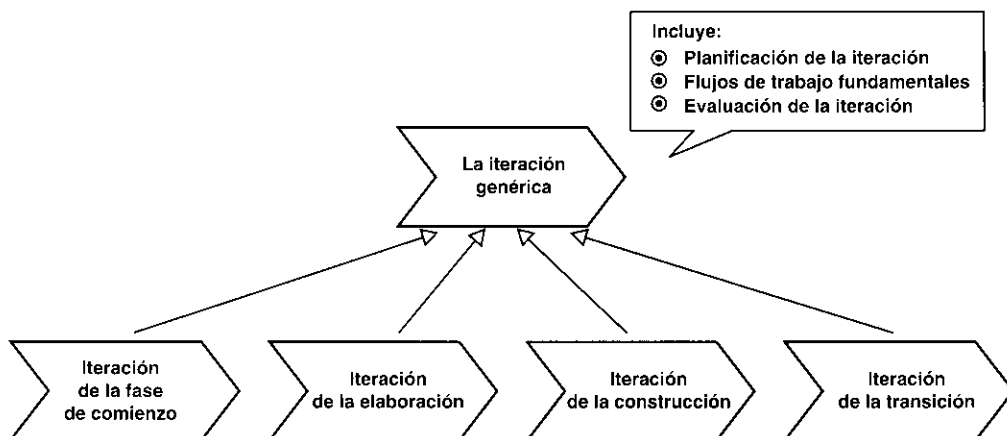
Figura 12.1. El flujo de trabajo de iteración genérica se emplea para describir los flujos de trabajo de iteración concretos para cada fase. (La intención de esta figura es ilustrar la forma en la que hemos estructurado la Parte III, con las generalidades sobre la iteración en el Capítulo 12 y las especializaciones para cada fase en los Capítulos 13-16).
