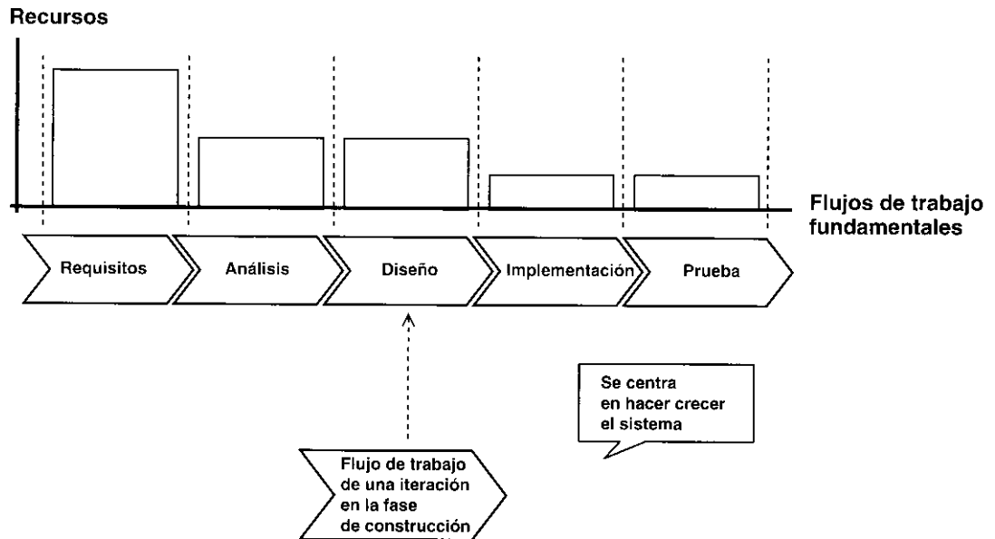
Figura 15.1. El trabajo de una iteración durante la fase de construcción discurre a lo largo de los cinco flujos de trabajo —requisitos, análisis, diseño, implementación y pruebas. Aquí se detallan y analizan los requisitos restantes, pero la carga de trabajo en estos dos flujos es relativamente leve. La mayor parte de este trabajo fue realizada en las dos fases anteriores. El diseño juega un papel importante, y es en esta fase en la que tiene lugar la mayor parte del trabajo de los flujos de implementación y pruebas. (El tamaño de las barras tiene un carácter meramente ilustrativo, y será distinto en diferentes proyectos.)
