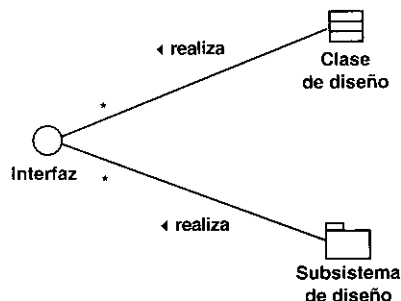
Figura 9.9. Las asociaciones fundamentales de una interfaz.
