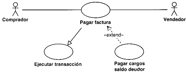
Figura 7.23. La relación de extensión entre los casos de uso Pagar Factura y Pagar Cargos Saldo Deudor.
