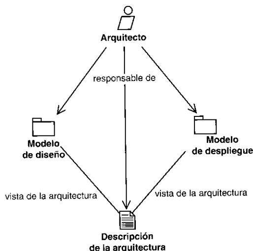
Figura 9.13. Las responsabilidades del arquitecto en el diseño.
