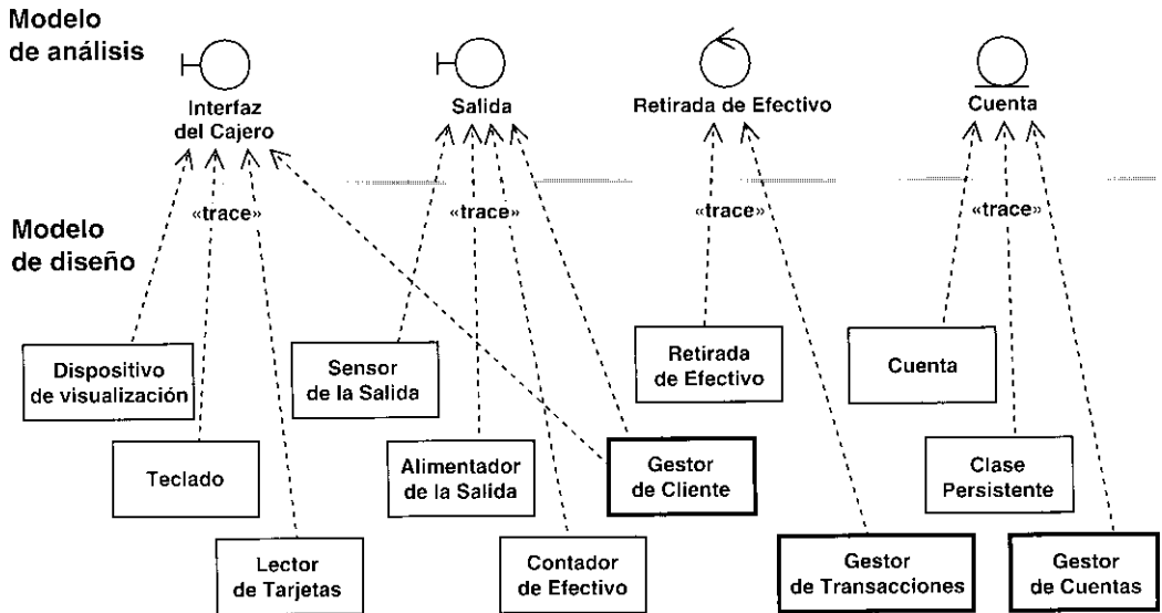
Figura 3.8. Clases de diseño del modelo de diseño con sus trazas hacia clases del modelo de análisis.
