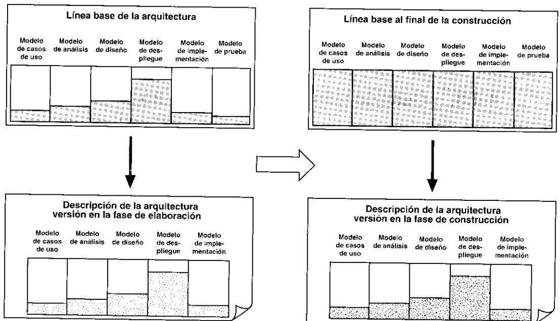
Figura 4.6. Durante la construcción, los diversos modelos van creciendo hasta completarse (según se muestra con las formas rellenas en la esquina superior derecha). La descripción de la arquitectura, sin embargo, no crece significativamente (abajo a la derecha) debido a que la mayor parte de la arquitectura se definió durante la fase de elaboración. Se incorporan pocos cambios secundarios a la arquitectura (indicados por un relleno punteado).
