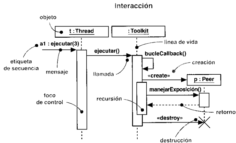
Figura A.5. Interacciones.
