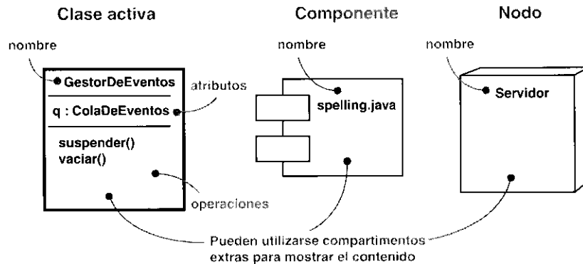
Figura A.4. Clases activas, componentes y nodos.
