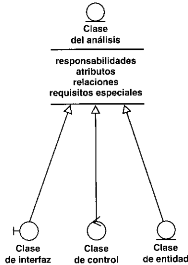
Figura 8.4. Los atributos esenciales y los subtipos (es decir estereotipos) de una clase del análisis.
