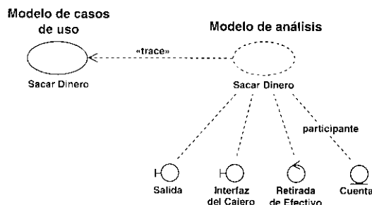
Figura 3.4. Las clases de análisis que participan en la realización de Sacar Dinero. Salida e Interfaz del Cajero son clases de interfaz, Retirada de Efectivo es una clase de control, y Cuenta es una clase de entidad.
