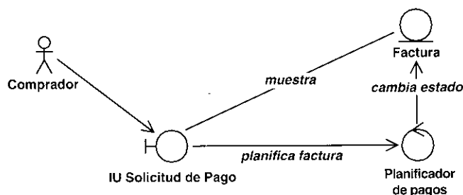
Figura 8.8. La clase de control planificador de pagos y sus relaciones con las clases de interfaz y de entidad.
